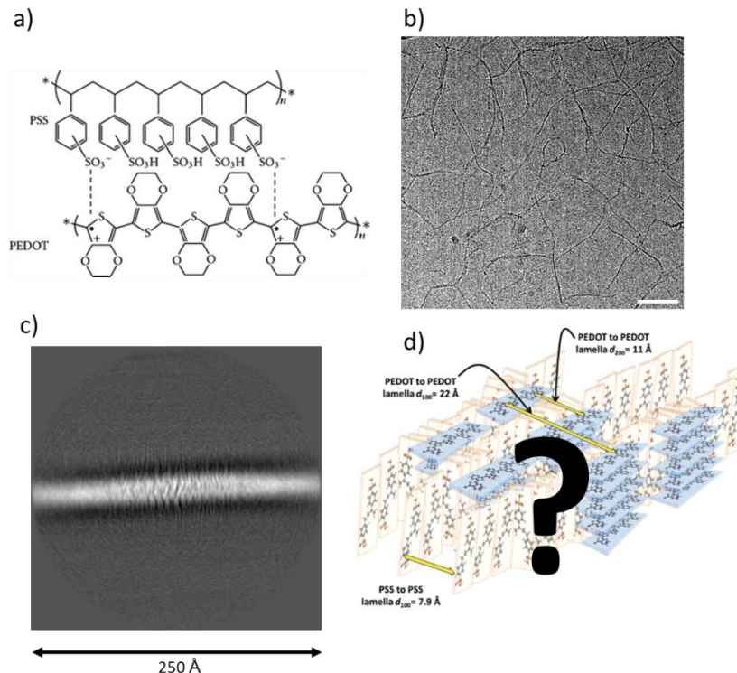
Figure 1 : a) Structure chimique du PEDOT :PSS, b) Image TEM en haute résolution (0.9 Å/pix) de la dispersion, c) une première classification 2D avec l'apparition d'un motif au centre et d) une potentielle structure proposée par Hosseini et al. 4
